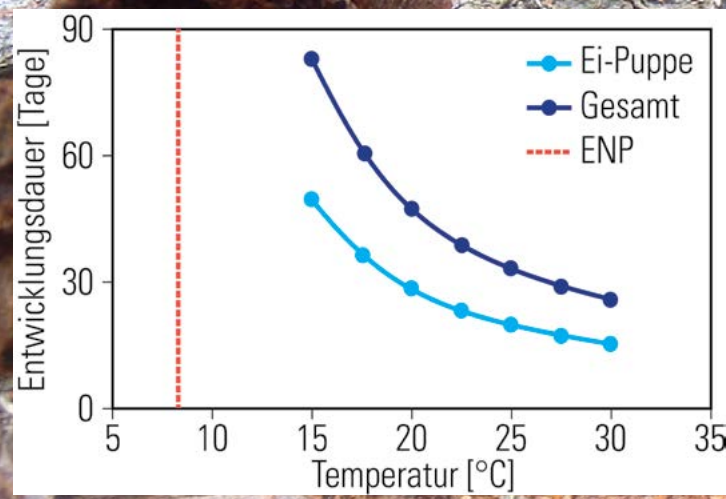
Buchdrucker - Entwicklungsdauer in Abhängigkeit von der Temperatur (ENP: Entwicklungsnullpunkt); Grafik: Hoch (BFW) nach Werminger und Seiffert 1998 bzw. Baier et al. 2007
